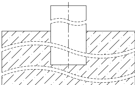
Установка столба без фланца в бетонное основание.
