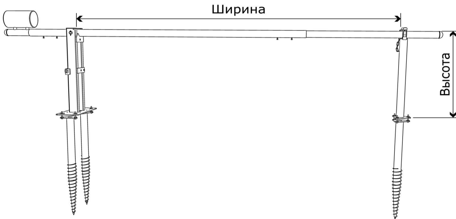
Внешний вид шлагбаума механического на примере арт. SH-0201 (с винтовыми опорами).
