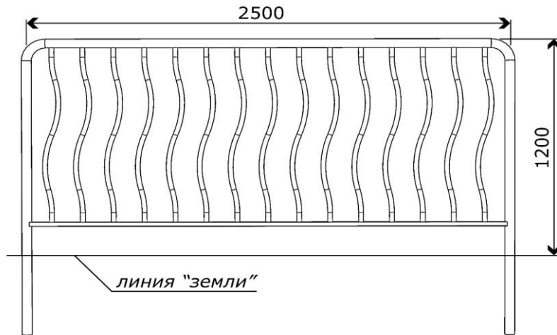
Эскиз ограждения без фланцев (PDS-27120)
