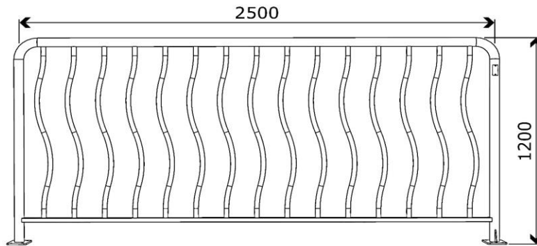
Эскиз ограждения с фланцами (PDS-27110)
