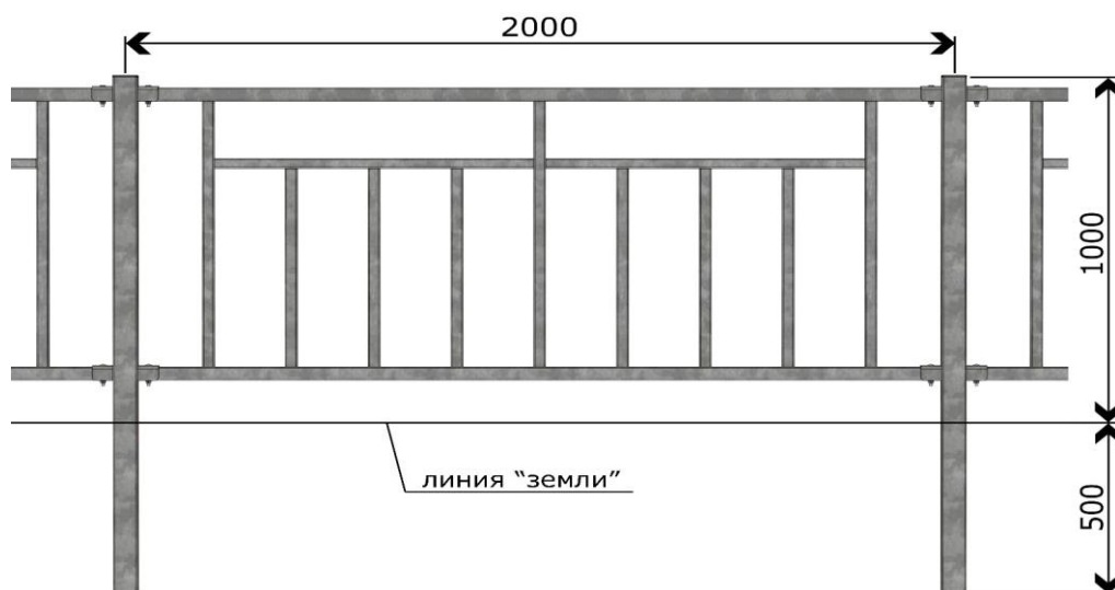
Эскиз ограждения без фланцев (стойка PDS-29110)
