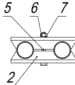
Б-Б (1:5)
