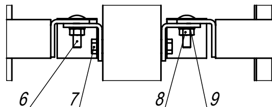
B (1 : 4) ☉
