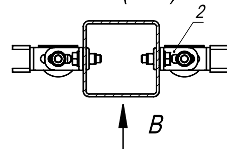
Б-Б (1 : 4)
