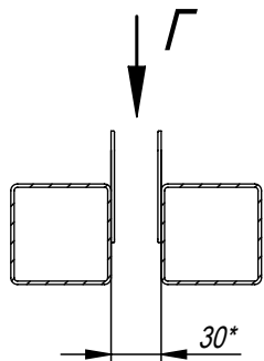
Б-Б (1:5)
