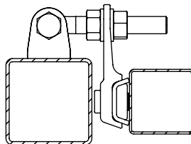
В-В (1:5)
