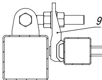
В-В (1:5)
