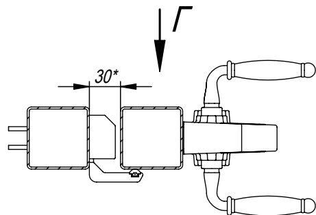
Б-Б (1:5)
