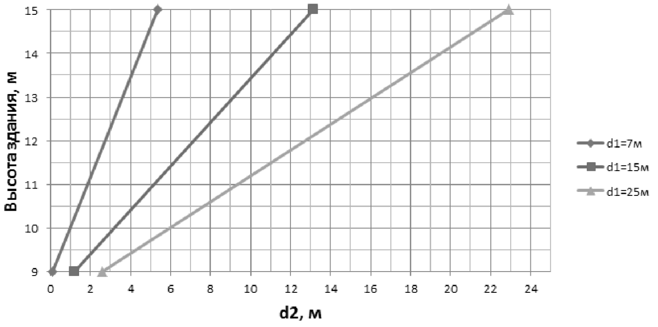
Зависимость между высотой здания Нзд и расстоянием d2 от него до ограждения высотой 8м
