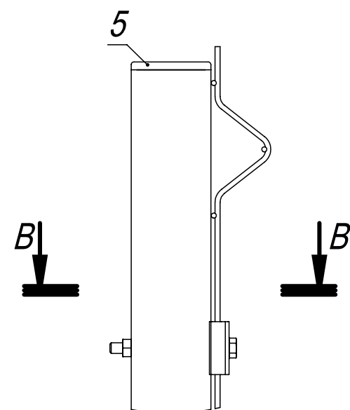
Б (1 : 4)
