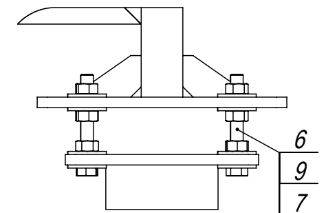
Г (1 : 5)
