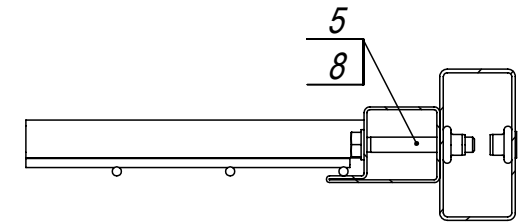
Б-Б (1 : 4)
