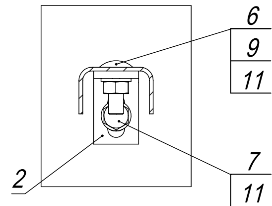
Б-Б (1 : 2)
