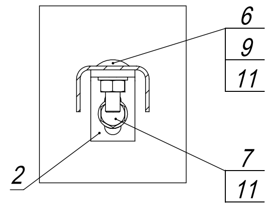
Б-Б (1 : 2)
